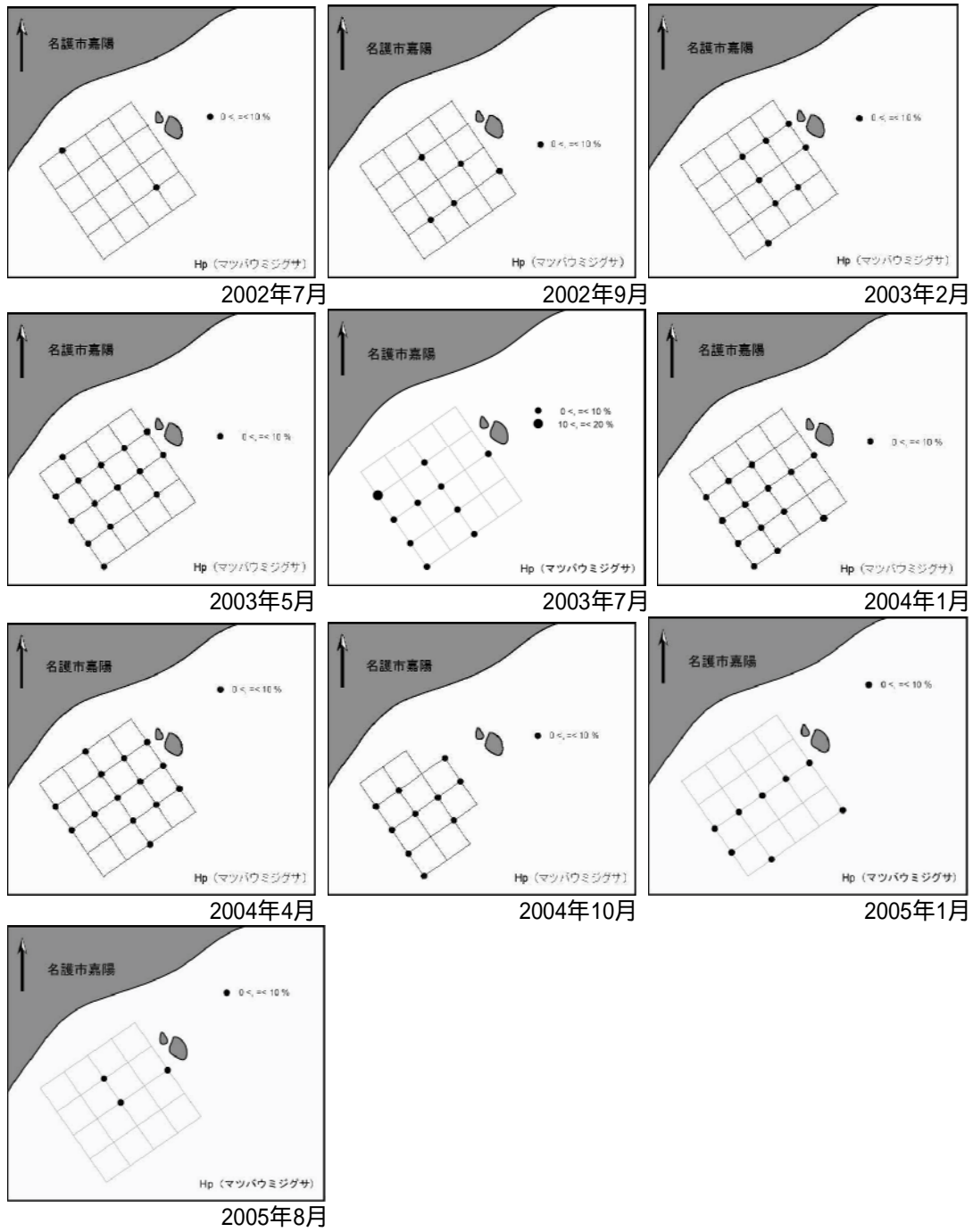
図14. 嘉陽におけるマツバウミジグサの分布
