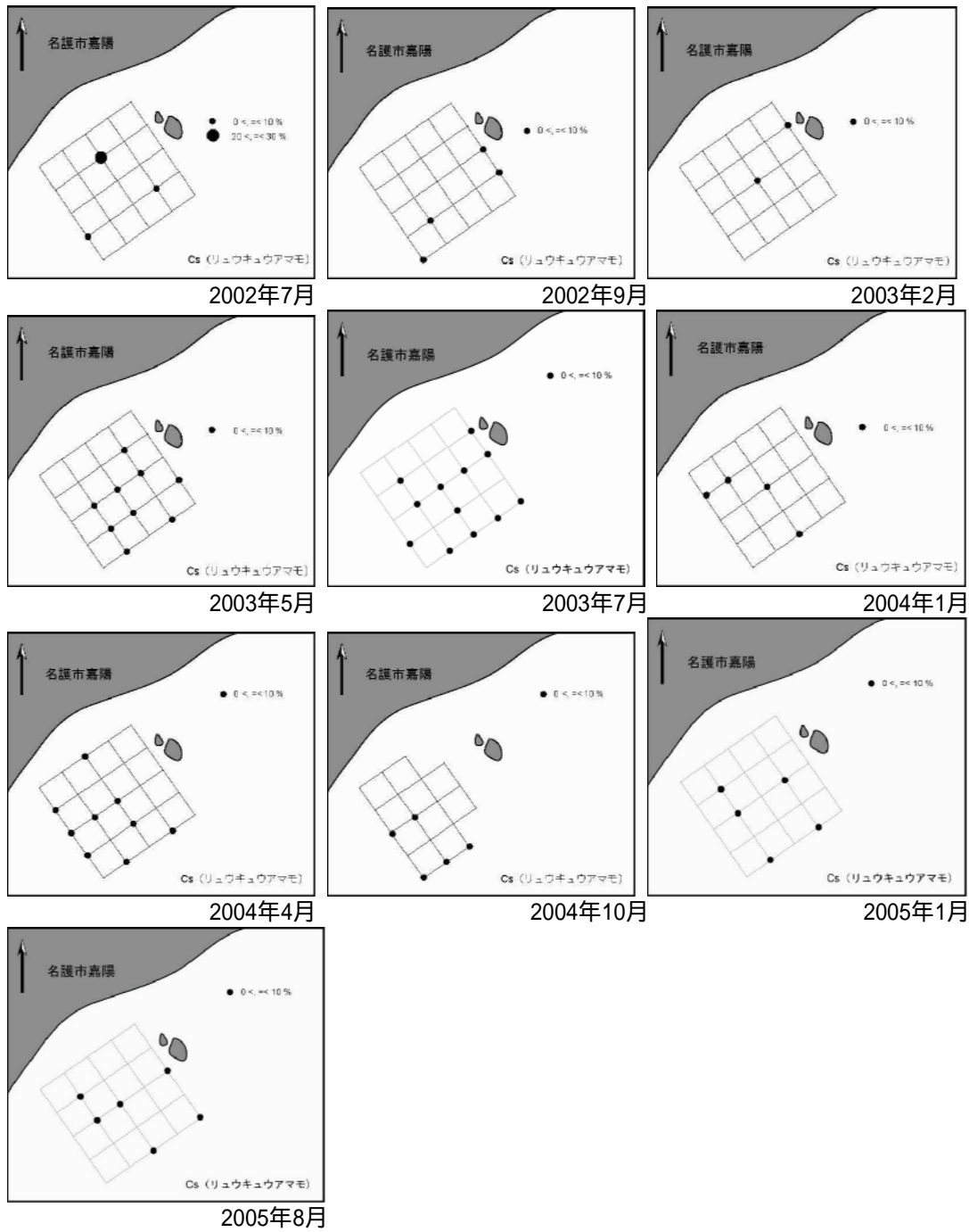
図11. 嘉陽におけるリュウキュウアマモの分布
