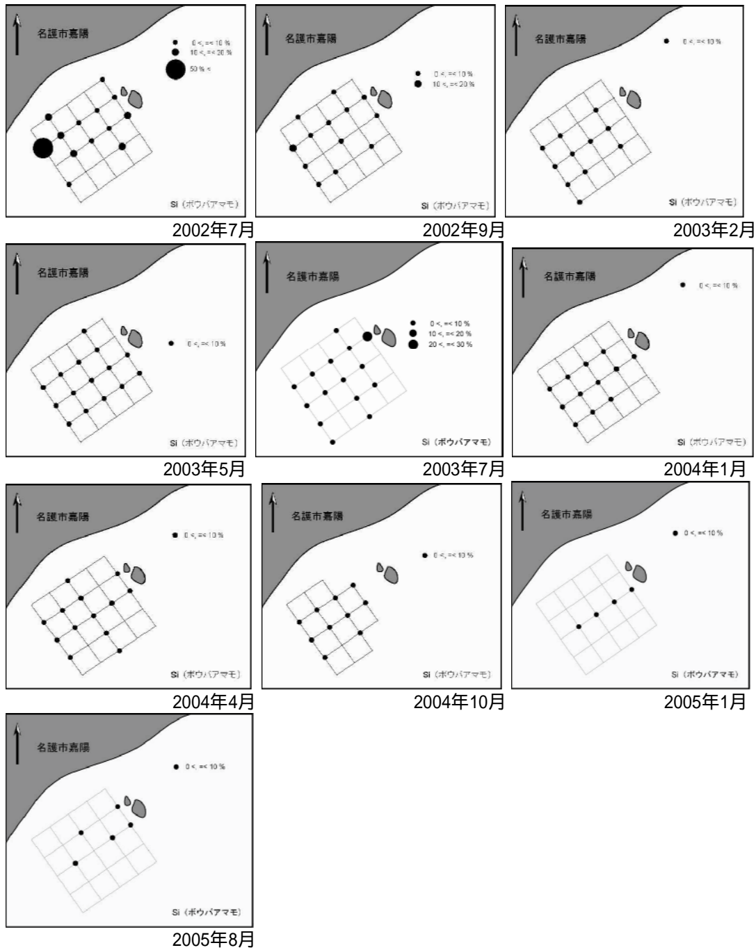
図8. 嘉陽におけるボウバアマモの分布
