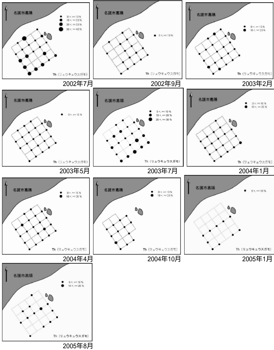
図9. 嘉陽におけるリュウキュウスガモの分布
