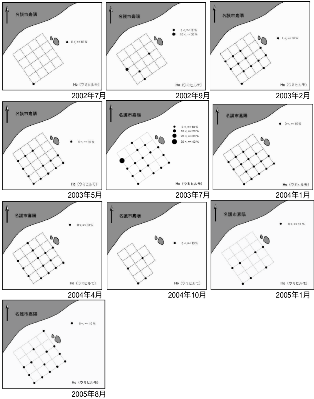
図10. 嘉陽におけるウミヒルモの分布
