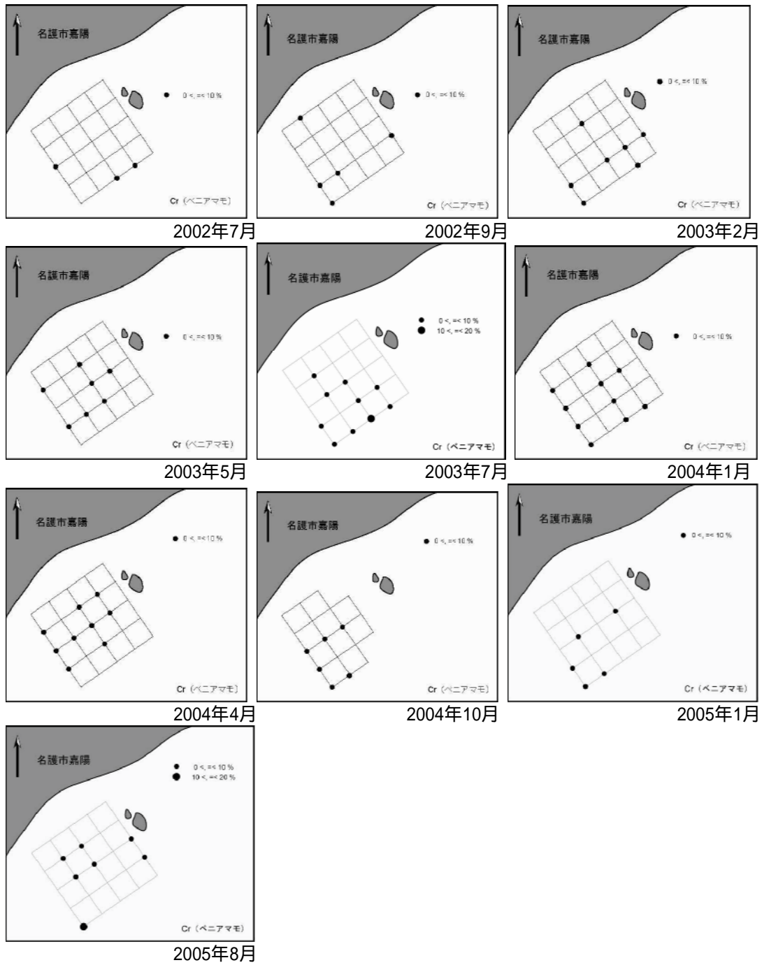
図12. 嘉陽におけるペニアマモの分布
