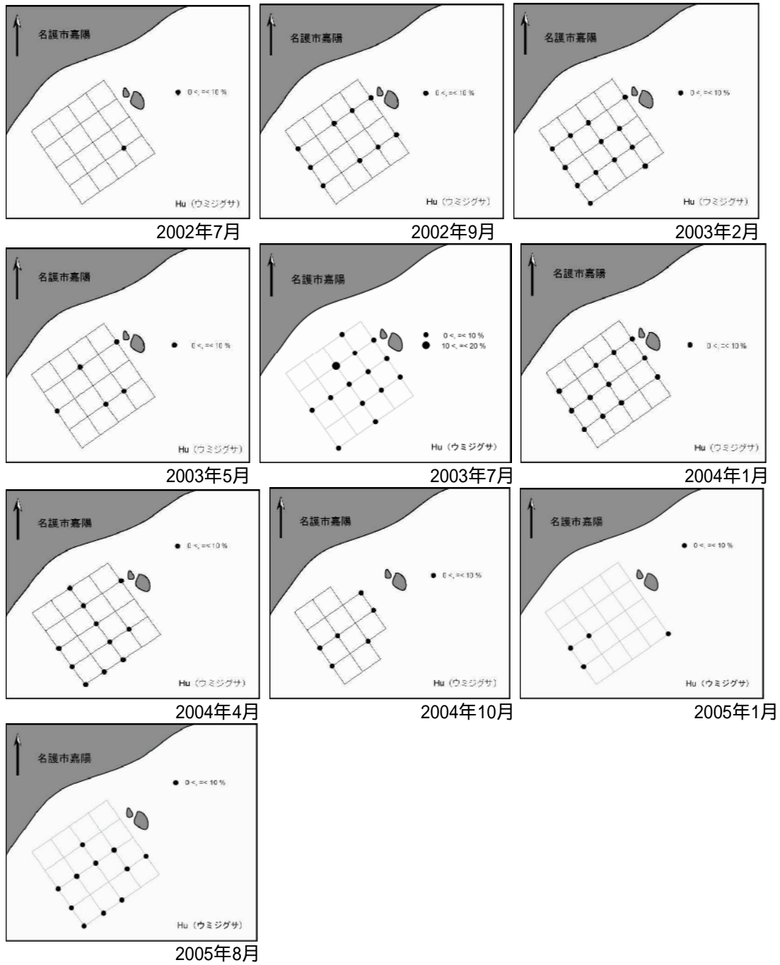
図13. 嘉陽におけるウミジグサの分布
