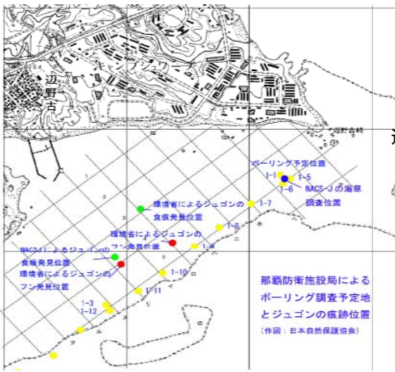
図 25. ジュゴンの痕跡の発見位置 とボーリング予定場所
