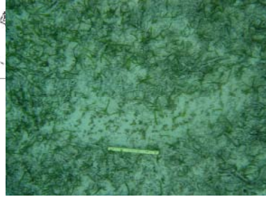
辺野古におけるジュゴンの食痕 (2004年1月)
