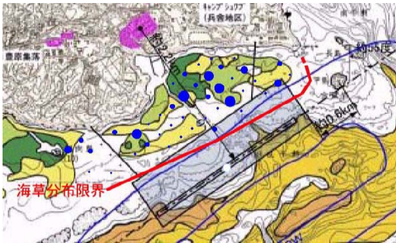
図 26. 辺野古における海草の 分布限界と空港計画 (防衛庁資料を改図)
